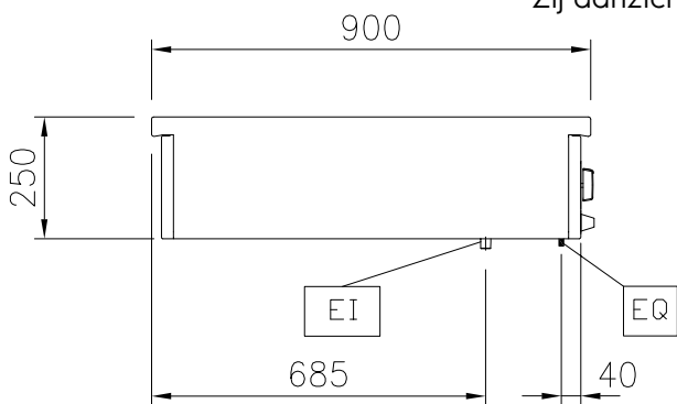
Zij aanzicht
